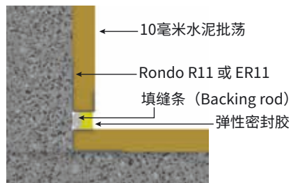
控制接缝拐角细节
