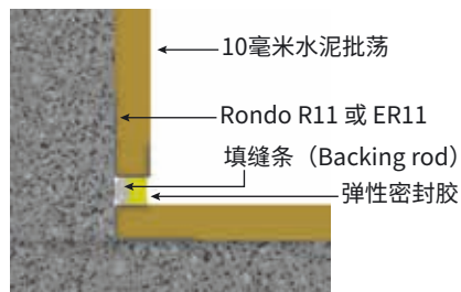
控制接缝拐角细节
